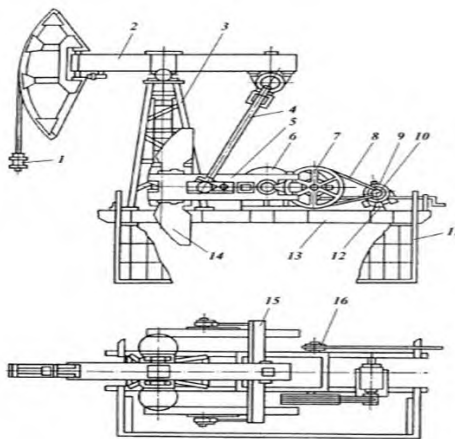
Рис. 5.2. Станок-качалка типа СК: 1 – подвеска устьевых штоков; 2 – балансир с опорой; 3 – стойка; 4 – шатуны; 5 – кривошипы; 6 – редуктор; 7 – ведомый шкив; 8 – ремень; 9 – электродвигатель; 10 – ведущий шкив; 11 – ограждение; 12 – поворотная плита; 13 – рама; 14 – противовес; 15 – траверса; 16 – тормоз
