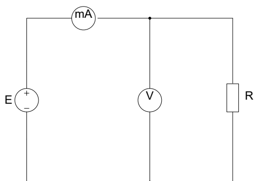
Рис. 1. Электрическая цепь постоянного тока
