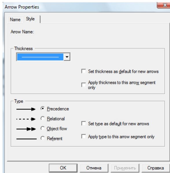
Рис. 3.5. Вкладка Style диалога Arrow Properties
