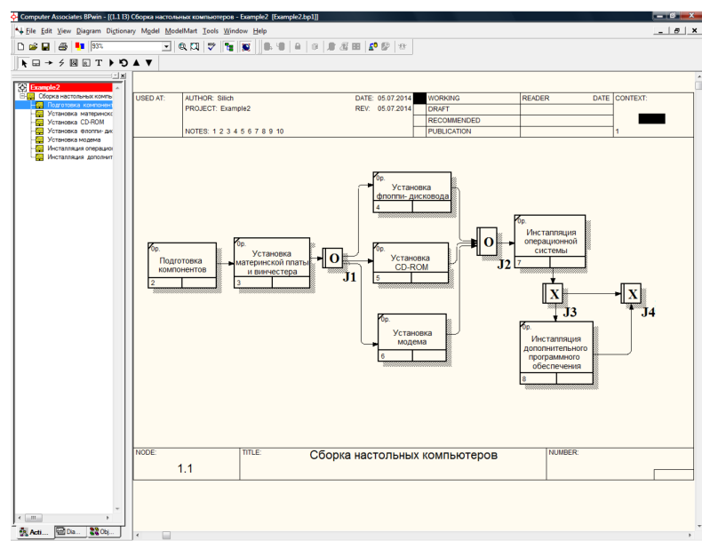
Рис. 3.6. Декомпозиционная диаграмма с перекрестками
