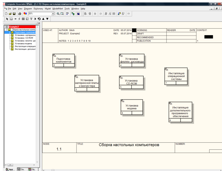
Рис. 3.4. Декомпозиционная диаграмма с функциональными блоками
