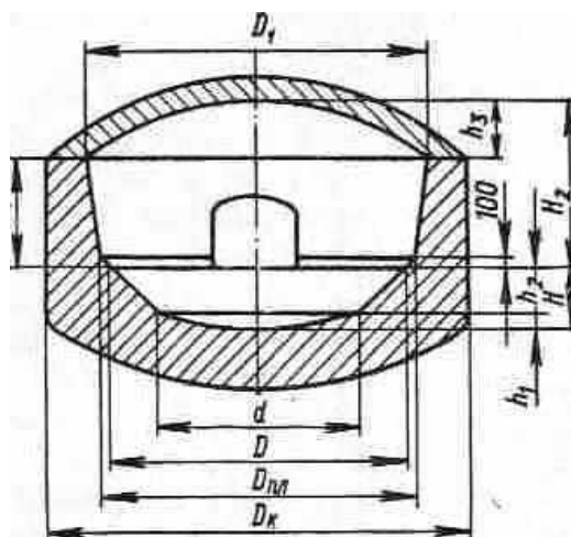
Рис. Форма плавильного пространства дуговой печи
