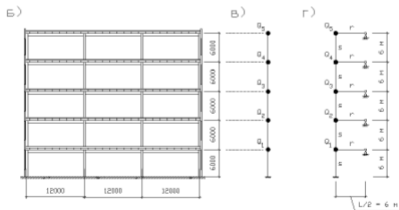
Рис. Схема многоэтажного здания.
