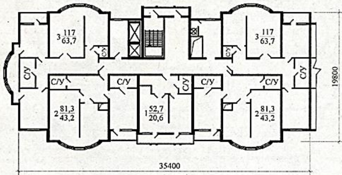
Типовой этаж
