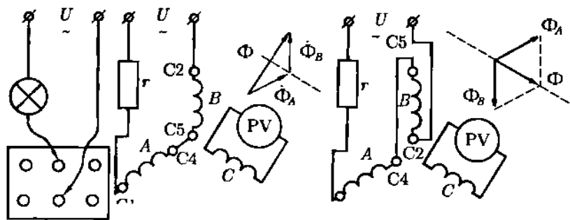
Рис. 1.1. Схемы для определения и маркировки выводов фазных обмоток статора.
