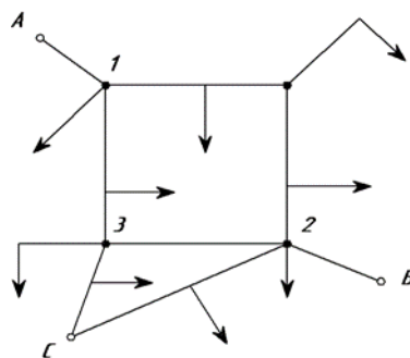
Рис. Схема сложной замкнутой сети Лабораторная работа №6
