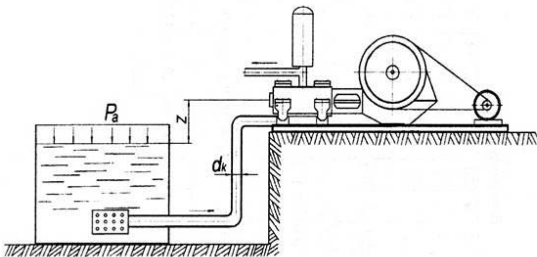
Схема установки насоса
