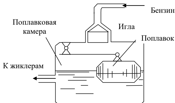
Рис. 1. Принципиальная схема регулирования уровня топлива в поплавковой камере.
