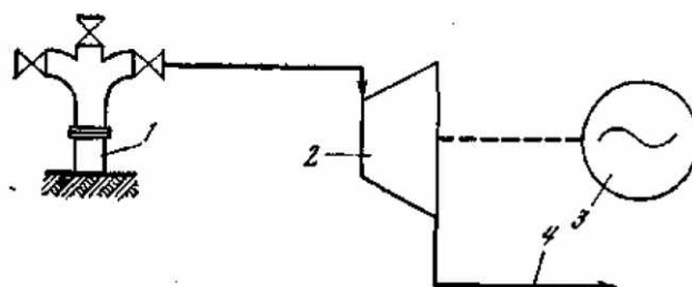
Рис. 1. Схема геотермальной электростанции с непосредственным использованием природного пара.
