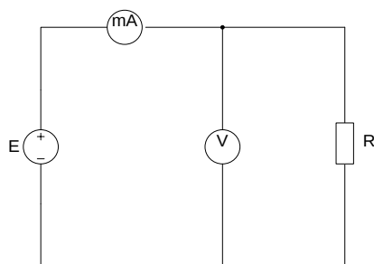
Рис. 1. Электрическая цепь постоянного тока
