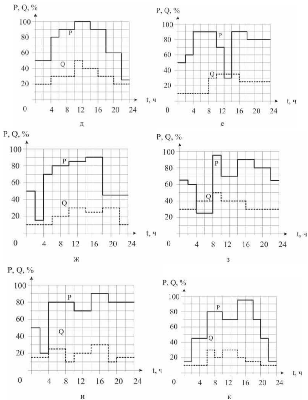
Рис.1 Суточные графики электрических нагрузок
