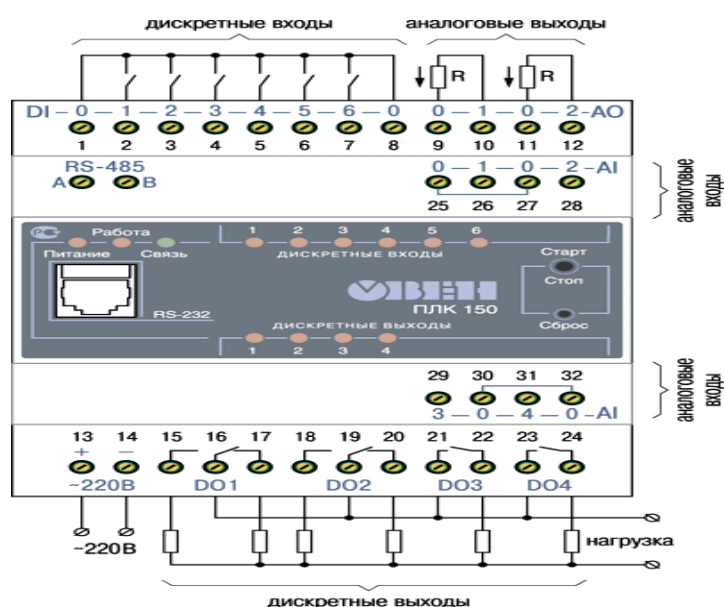
Рис.1. Схема подключения внешних соединений ПЛК150-220
